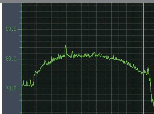
Geräuschemission bei Verwendung von Super8
