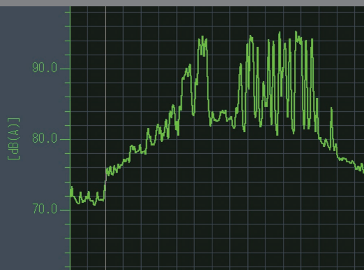
Geräuschemission bei Verwendung von herkömmlichen Sägeband
